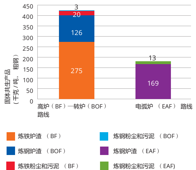
钢铁生产路线产生的主要固体共生产品 2 (平均产量 千克 / 吨 粗钢)
